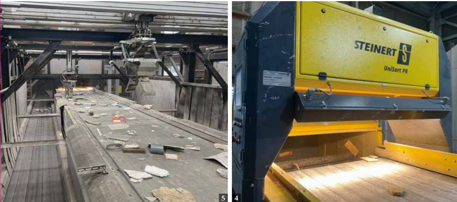
1.九州北部豪雨で活躍した移動式 破砕機とフルイ機。約1年半かけて 現地処理を完了させた/2.九州北部 豪雨で活躍した九州に一台しかない 車載型移動式選別機/3.見学通路 /4.近赤外線素材を認識・選別 する光化学式選別機/5.AIを搭載 した選別ロボット/6.4種類のセン サー(カラー、金属探知、近赤外線、 画像)を活用し、廃棄物を素材で認識 している
